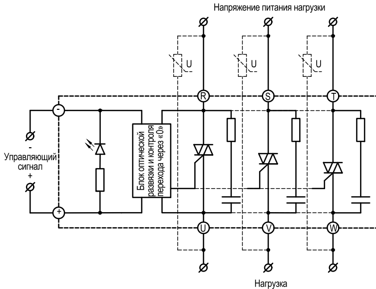
Рисунок 30 – схема подключения ТТП серии HT-●●44.ZD3 ( \leq 40 А)
