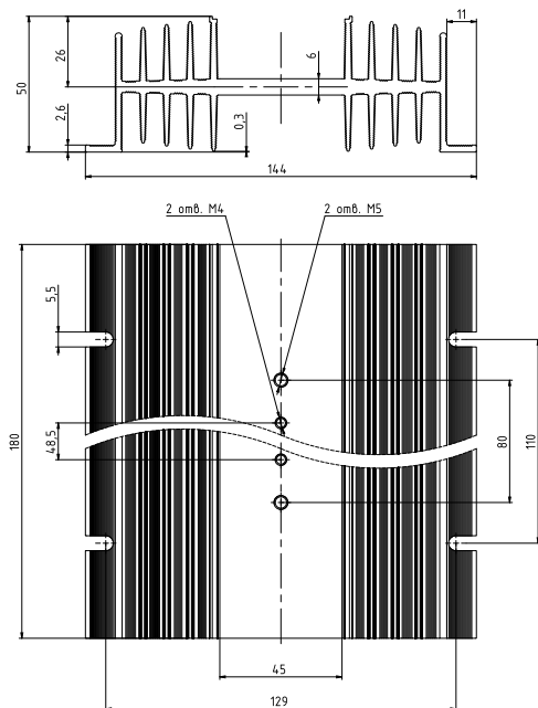
Рисунок 53 – габаритные и установочные размеры радиатора PTP063.1
