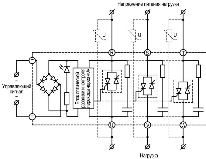
Рисунок 34 – схема подключения ТТР серии HT-●●44.ZA2 ( \geq 60 А)
