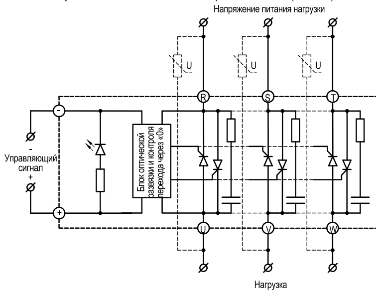
Рисунок 32 – схема подключения ТТР серии HT-●●44.ZD3 ( \geq 100 A)
