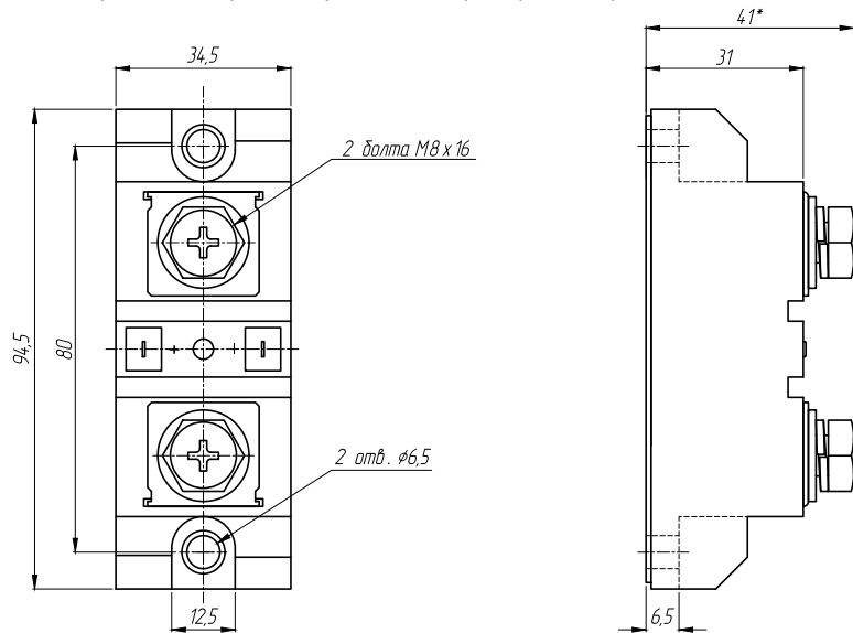
Рисунок 22 – габаритные и установочные размеры ТТР серии BDH-●●44.ZD3
