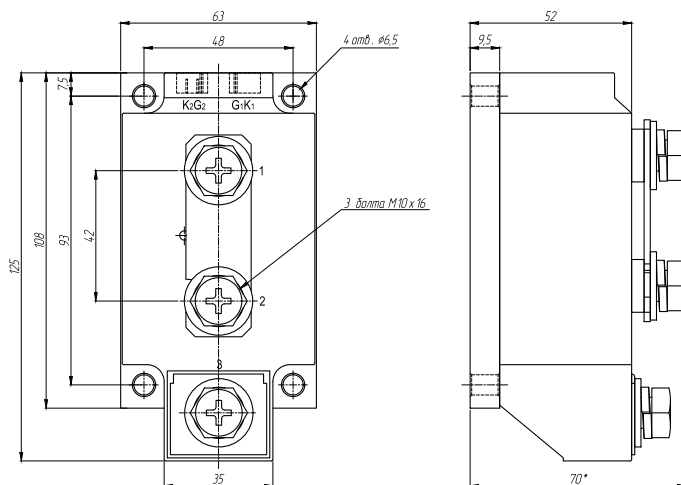
Рисунок 25 – габаритные и установочные размеры ТТП серии GaDH-800120.ZD3
