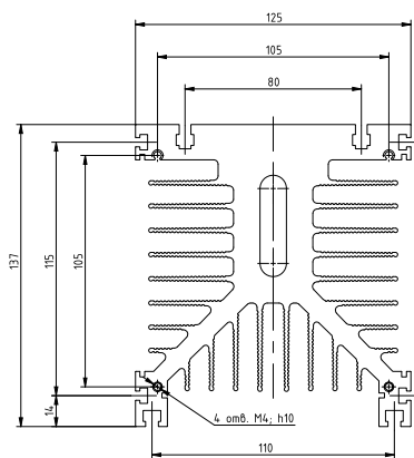
Рисунок 59 – габаритные и установочные размеры радиатора PTP040
