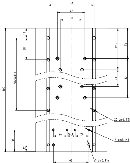
Рисунок 59 – габаритные и установочные размеры радиатора PTP040
