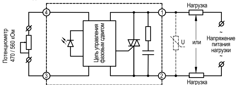
Рисунок 16 – схема подключения ТТР серии HD-●●44.VA
