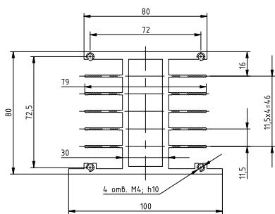
Рисунок 55 – габаритные и установочные размеры радиатора РТР036
