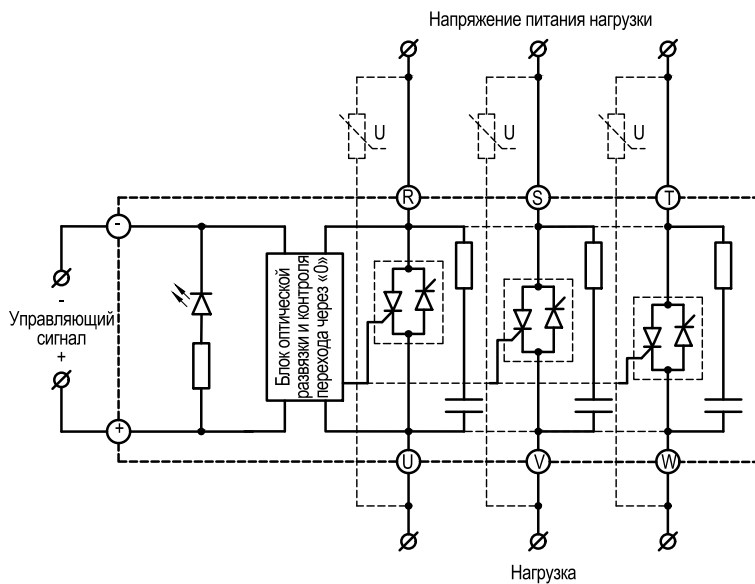
Рисунок 31 – схема подключения ТТР серии HT-●●44.ZD3 (60 и 80 A)
