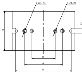
Рисунок 50 – габаритные и установочные размеры радиатора PTP060
