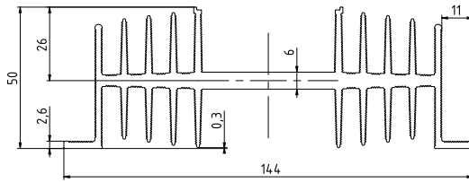
Рисунок 50 – габаритные и установочные размеры радиатора PTP060
