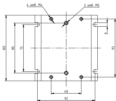
Рисунок 54 – габаритные и установочные размеры радиатора РТР034
