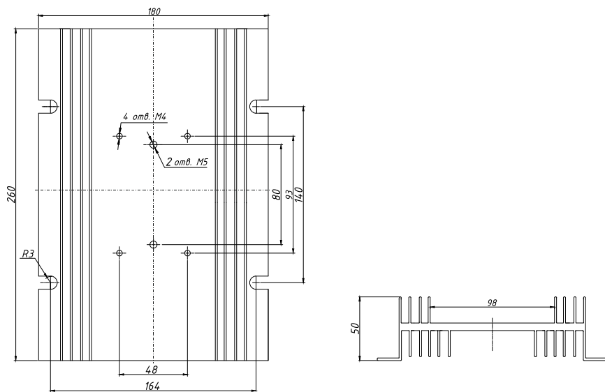
Рисунок 56 – габаритные и установочные размеры радиатора РТР037
