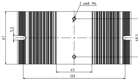
Рисунок 51 – габаритные и установочные размеры радиатора PTP061.1
