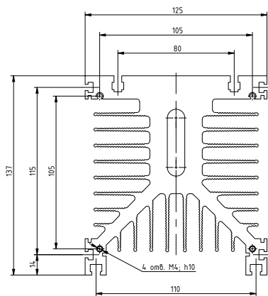
Рисунок 58 – габаритные и установочные размеры радиатора PTP039
