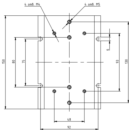
Рисунок 55 – габаритные и установочные размеры радиатора РТР036
