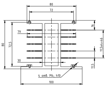
Рисунок 54 – габаритные и установочные размеры радиатора РТР034
