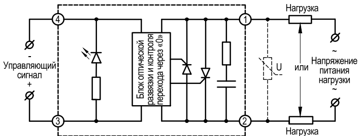
Рисунок 20 – схема подключения ТТП серии HDH-●●44.ZD3
