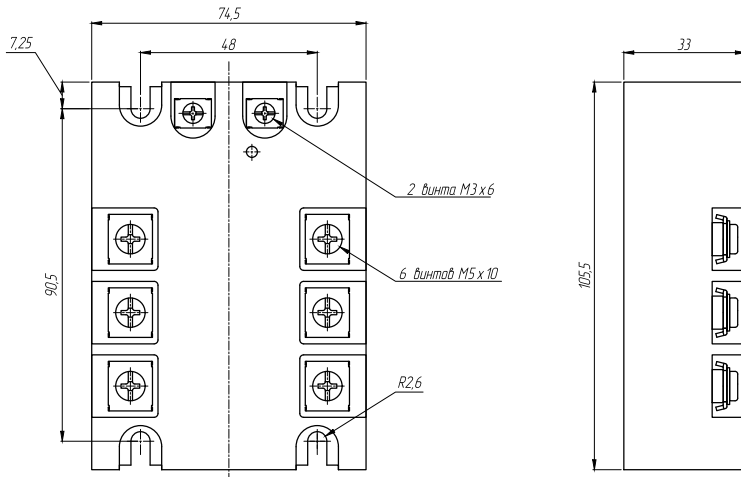
Рисунок 29 – габаритные и установочные размеры ТТП серий HT-●●44.ZD3 / ZA2
