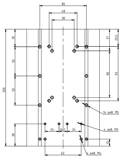
Рисунок 58 – габаритные и установочные размеры радиатора PTP039
