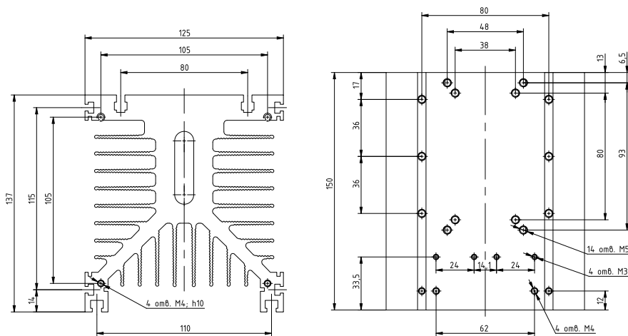
Рисунок 57 – габаритные и установочные размеры радиатора РТР038
