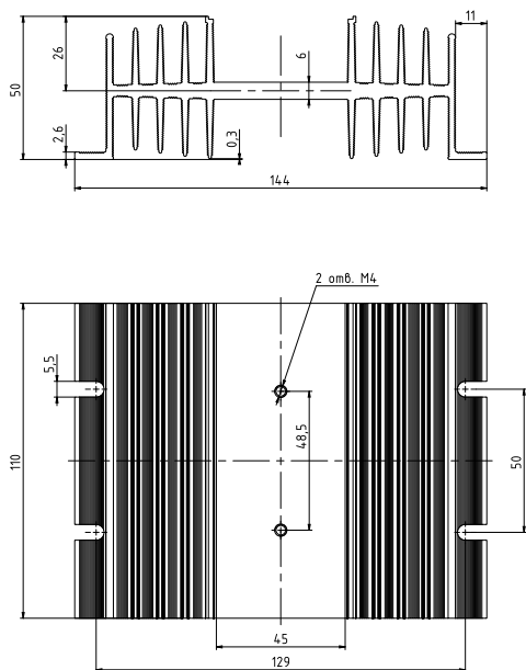
Рисунок 52 – габаритные и установочные размеры радиатора PTP062.1
