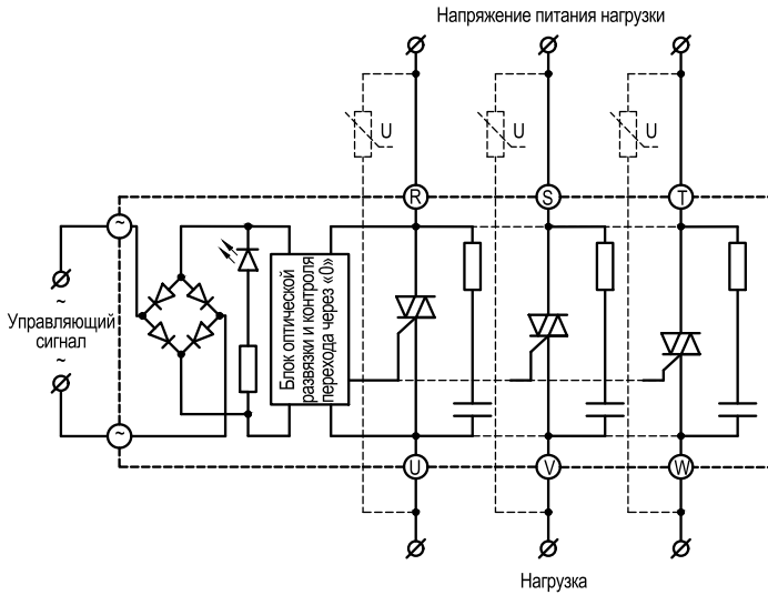
Рисунок 33 – схема подключения ТТР серии HT-●●44.ZA2 ( \leq 40 А)
