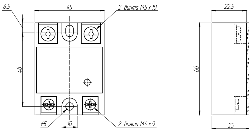
Рисунок 15 – габаритные и установочные размеры ТТП серии HD-●●22.10U
