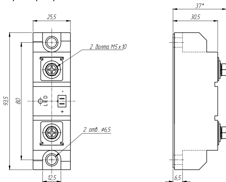
Рисунок 21 – габаритные и установочные размеры ТТР серии SBDH-●●44.ZD3
