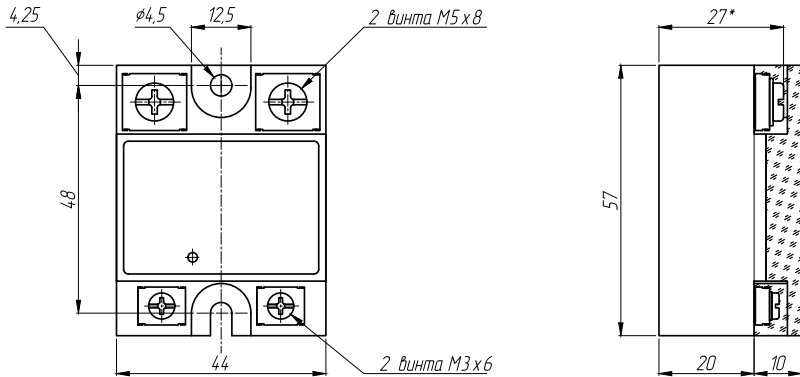
Рисунок 19 – габаритные и установочные размеры ТТП серии HDH-●●44.ZD3
